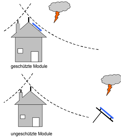
Module innerhalb des Blitzschutzes montieren
