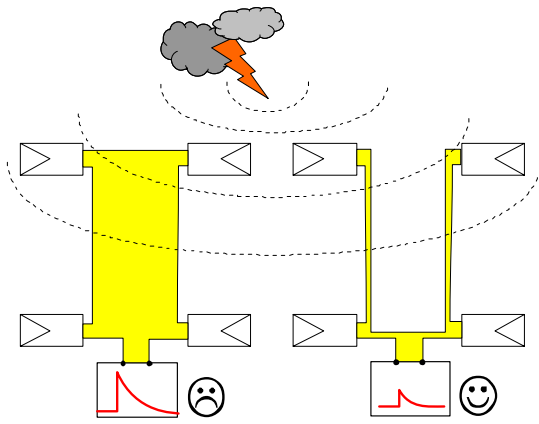
Schleifenbildungen vermeiden
