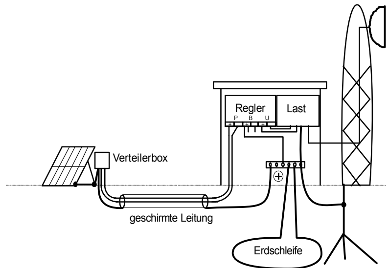
Module innerhalb des Blitzschutzes montieren
